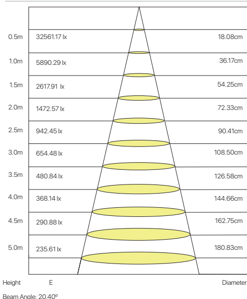
Lux, Curva de distancia
